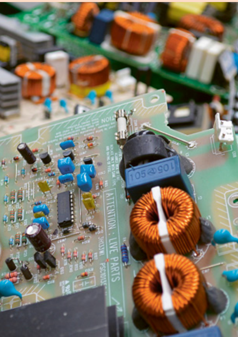
Les déchets électroniques et électriques : un gisement de ressources minérales stratégiques.
